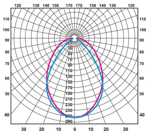
КСС светильника ЛВО418 М
