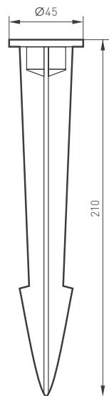
Рис. 1. Чертеж и габаритные размеры светильника
