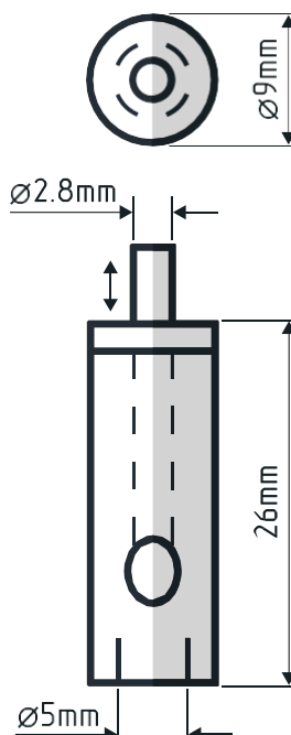
Зажим SKP012 1505232012
