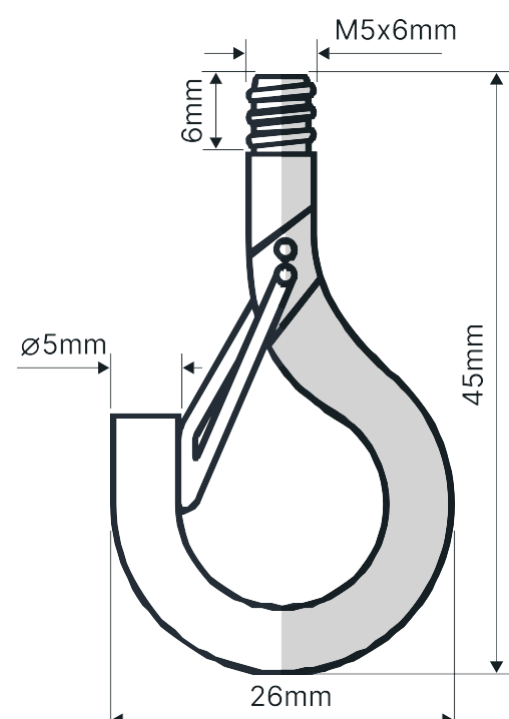
Крюк SKP014 1505232014
