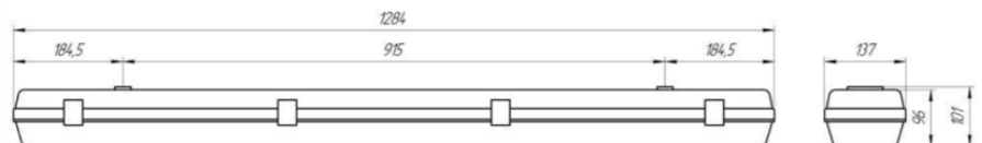
Схема проекции, размеры
