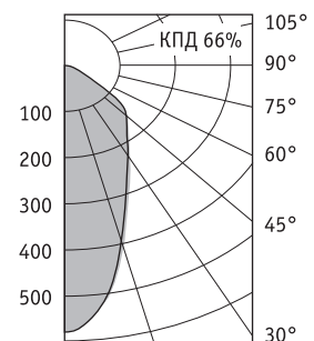
FHE/T HG70 (45°)
