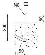
Комплект анкерных болтов АВ 160. Код заказа — 2407000010.
