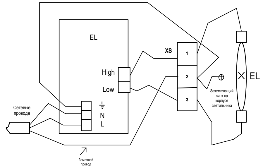
Схема электрическая светильника.
