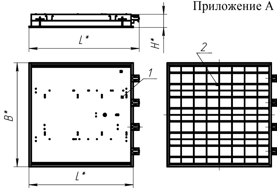
Рисунок 1.1. Корпус в сборе, 2. Решетка зеркальная.
