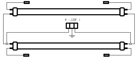
Рисунок 5.2 Схема подключения светильника ДВО10-2x22 с LED лампами
