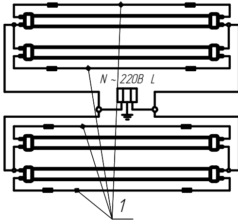
Рисунок 3. 1 Схема подключения ДВО10-4x11-004 с LED лампами типа PHILIPS.
