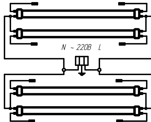
Рисунок 3. 2 Схема подключения ДВО10-4x11-004 с LED лампами .
