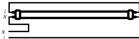
Рисунок 4. 1 Схема подключения LED ламп типа PHILIPS (тип 1).
