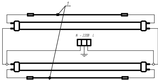
Рисунок 5.1 Схема подключения светильника ДВО10-2x22 с LED лампами типа PHILIPS
