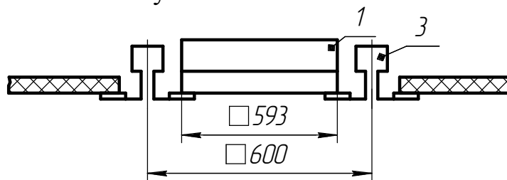
Рисунок 2. 1. Светильник в сборе, 3. Элемент подвесной системы потолка.
